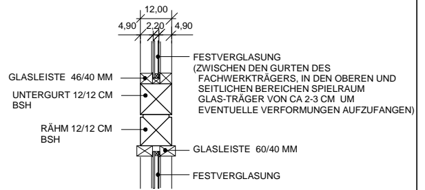
DETAIL J 1 M: 1/10
