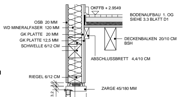
DETAIL K 1 M: 1/10
