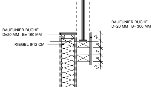
DETAIL H 3 M: 1/10
